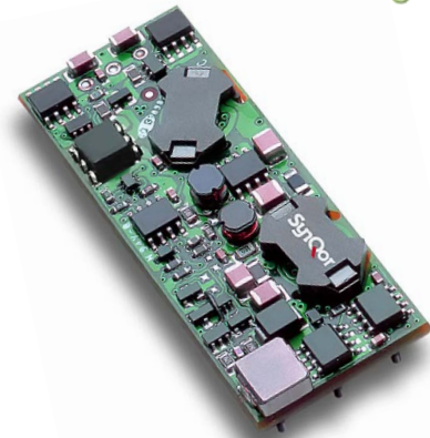
PQ60010EGL20 Module
